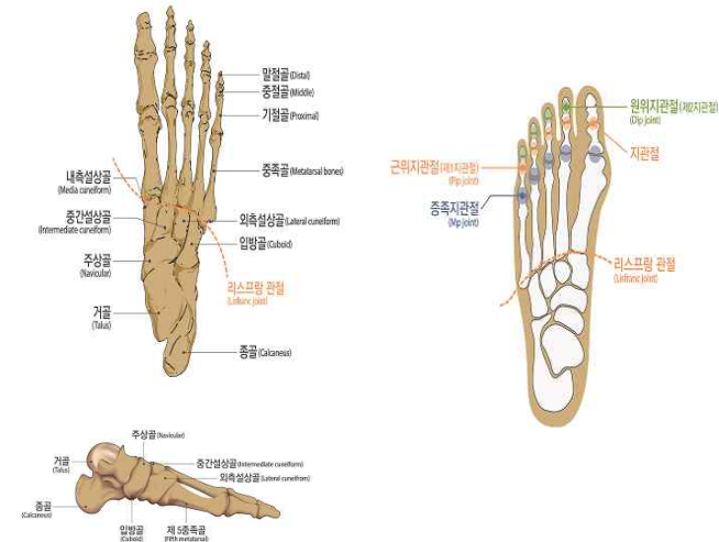
< 발가락 >
