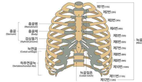
< 가슴뼈 >
